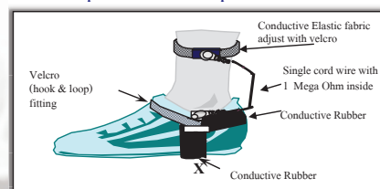
Heel Strap Model E
