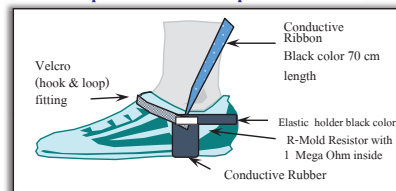
Heel Strap Model D
